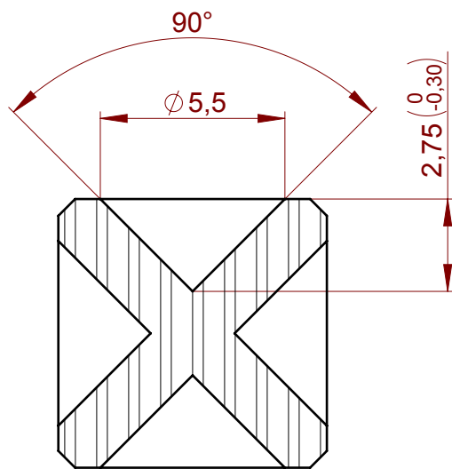
SEZIONE A-A SCALA 5 : 1
