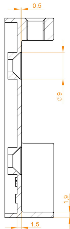
SEZIONE A-A
