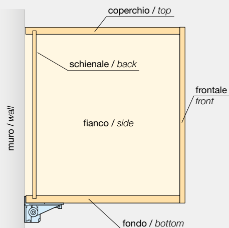
SEZ. / SECT.
