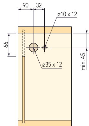
SEZ. / SECT.
