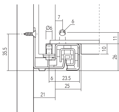
Schema di foratura / Drilling pattern
