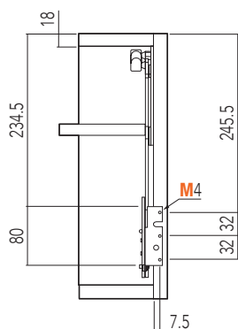
INT. FORATURA PER ANTA ALLUMINIO TELAIO 20x20 INNER PART OF THE HOLE FOR ALUMINIUM DOOR 20x20
