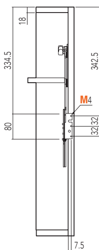
INT. FORATURA PER ANTA ALLUMINIO TELAIO 20x20 INNER PART OF THE HOLE FOR ALUMINIUM DOOR 20x20
