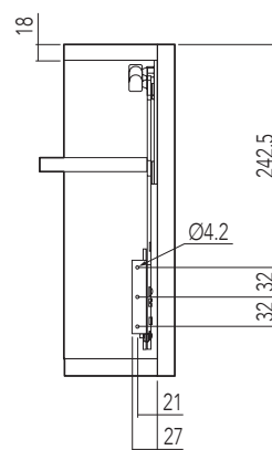
INT. FORATURA PER ANTA ALLUMINIO TELAIO 45x20 INNER PART OF THE HOLE FOR ALUMINIUM DOOR 45x20
