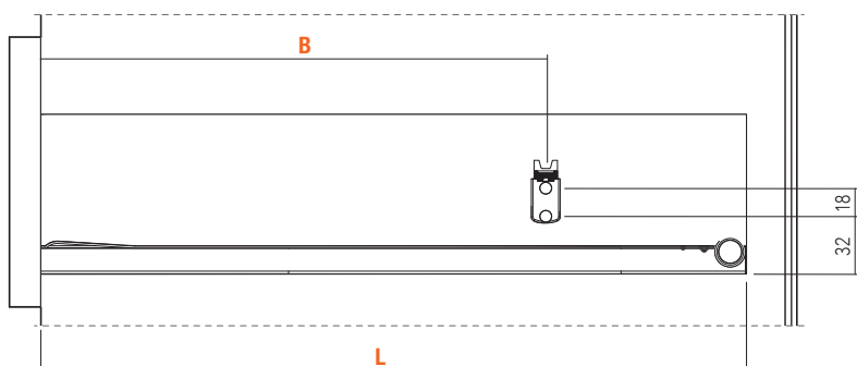
Fissaggio al cassetto / Drawers fixing method
