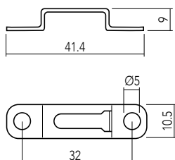
B clip aperta / open clip
