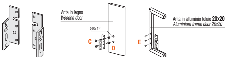
INT. FORATURA PER ANTA ALLUMINIO TELAIO 20x20 INNER PART OF THE HOLE FOR ALUMINIUM DOOR 20x20
