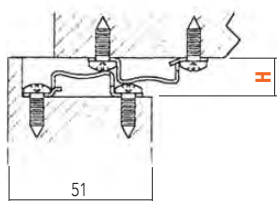
Scanalatura aperta / open pocket
