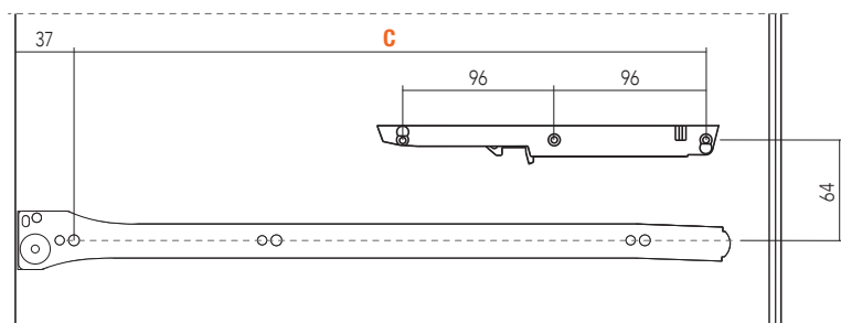
Schema di montaggio / Assembly
