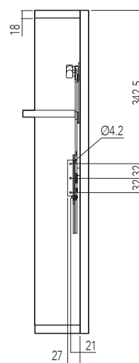
INT. FORATURA PER ANTA ALLUMINIO TELAIO 45x20 INNER PART OF THE HOLE FOR ALUMINIUM DOOR 45x20
