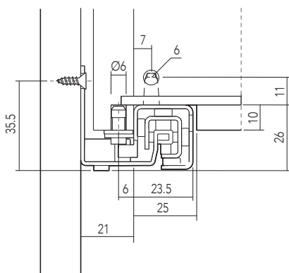
Schema di foratura / Drilling pattern
