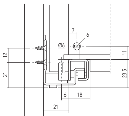
Schema di foratura / Drilling pattern
