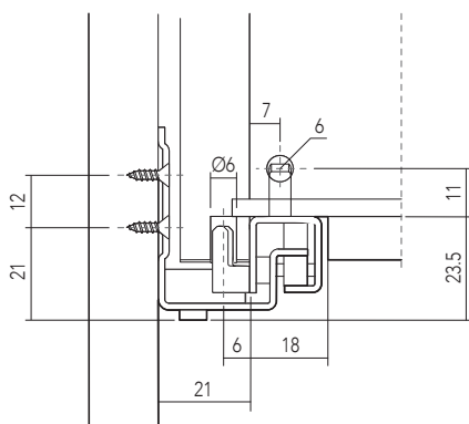
Schema di foratura / Drilling pattern
