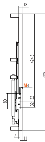
INT. FORATURA PER ANTA ALLUMINIO TELAIO INNER PART OF THE HOLE FOR ALUMINIUM DOOR
