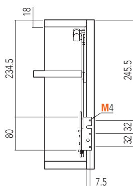
INT. FORATURA PER ANTA ALLUMINIO TELAIO 20x20 INNER PART OF THE HOLE FOR ALUMINIUM DOOR 20x20
