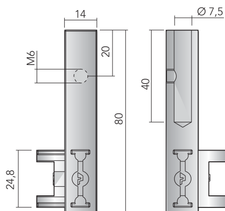
REGGITUBO ANGOLARE CORNER BRACKET
