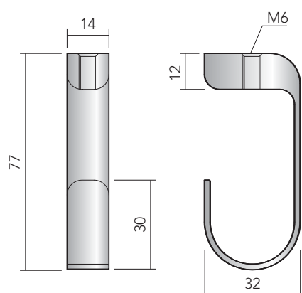
REGGITUBO CENTRALE CENTRAL BRACKET
