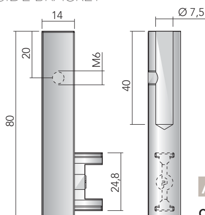
REGGITUBO LATERALE - SX SIDE BRACKET
