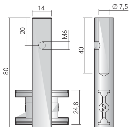
REGGITUBO CENTRALE CENTRAL BRACKET
