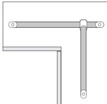
UTILIZZO IN ARMADI AD ANGOLO USE IN A CORNER WARDROBE
