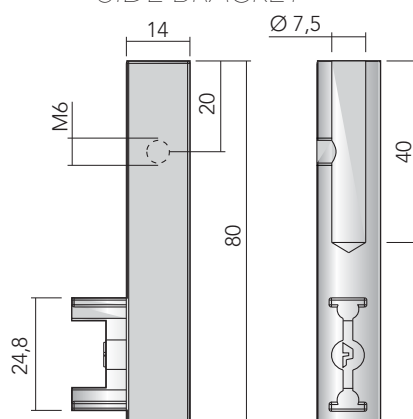
REGGITUBO LATERALE - DX SIDE BRACKET
